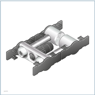
Longitudinal end connector
